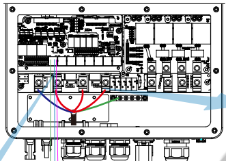
Вимикач змінного струму
