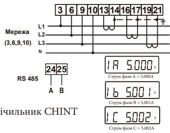
230/400В, 3~ 250А/50мА 50/60 Гц CHNT DTSU666
